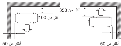
عرض علوي
