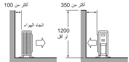
عرض جانبي
